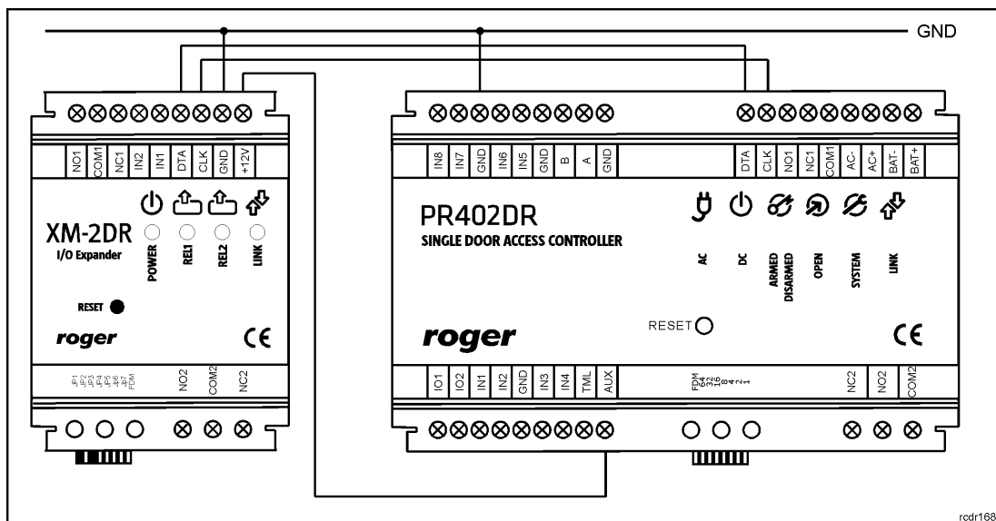
Rys. 2 Podłączenie moduły XM-2DR (ID=5) do kontrolera PR402DR
